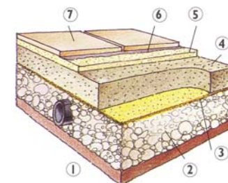
Chape isolante sous sol en terre cuite traditionnelle (doc. J.-P. Oliva).
