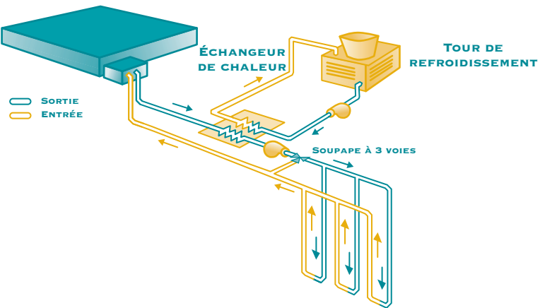
FIGURE 25. ÉVACUATEUR DE CHALEUR AUXILIAIRE – TOUR DE REFROIDISSEMENT
