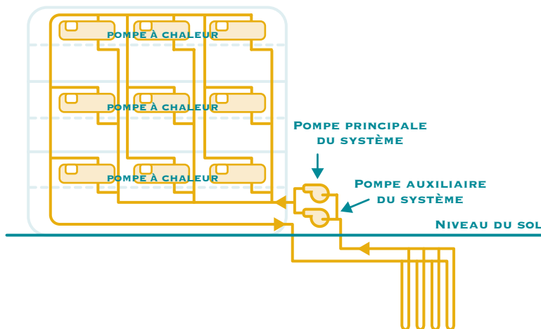
FIGURE 17. SYSTÈME DE DISTRIBUTION TYPIQUE DE SYSTÈME À BOUCLE DE SOL
