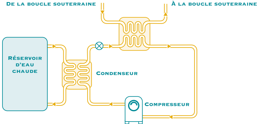
FIGURE 21. CHAUFFE-EAU À POMPE À CHALEUR
