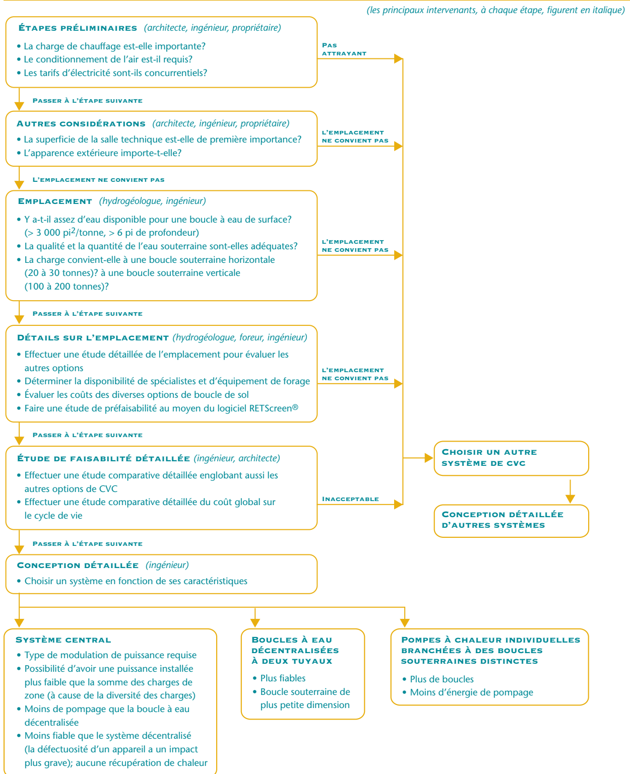
FIGURE 27. DÉROULEMENT TYPE D'UN PROJET DE SYSTÈME GÉOTHERMIQUE
