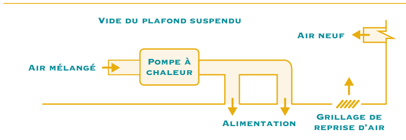
FIGURE 19. VIDE DU PLAFOND UTILISÉ COMME CAISSON D'AIR DE RETOUR
