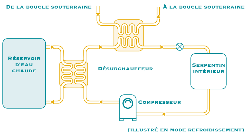
FIGURE 20. DÉSURCHAUFFEUR
