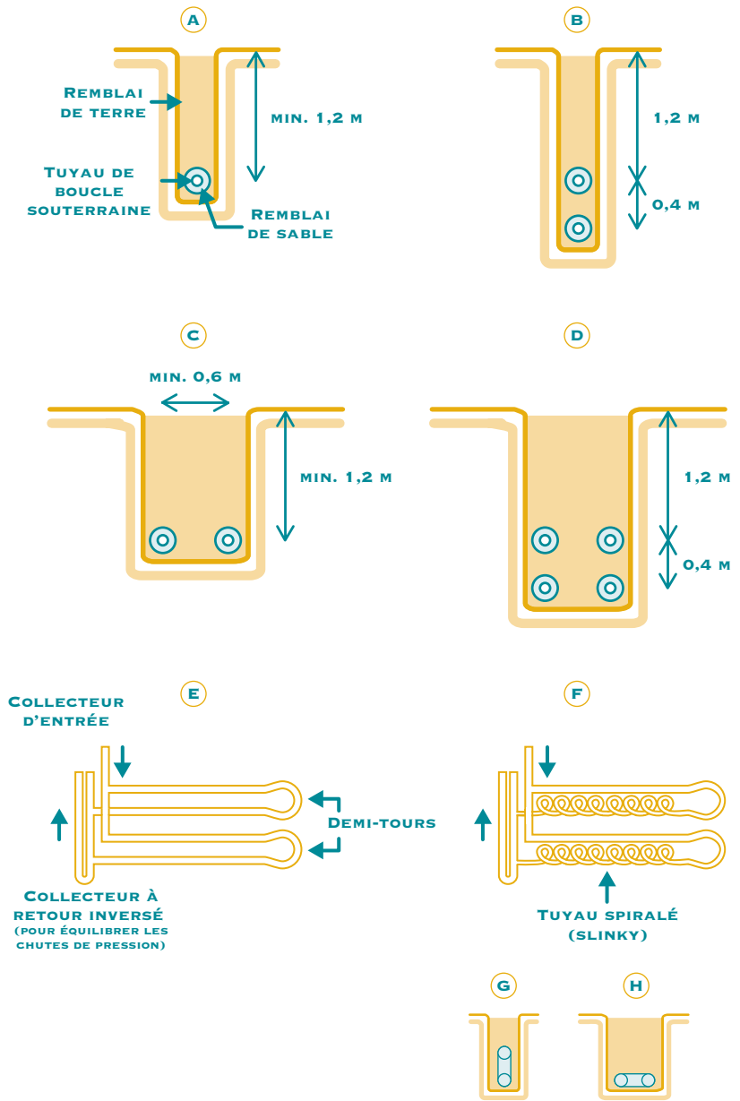
FIGURE 12. DIVERS TYPES DE BOUCLES HORIZONTALES
