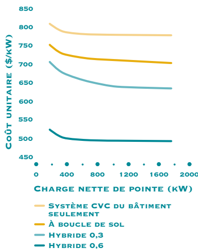
FIGURE 7. COÛT TYPE D'UN SYSTÈME À BOUCLE DE SOL ET DE SYSTÈMES HYBRIDES
