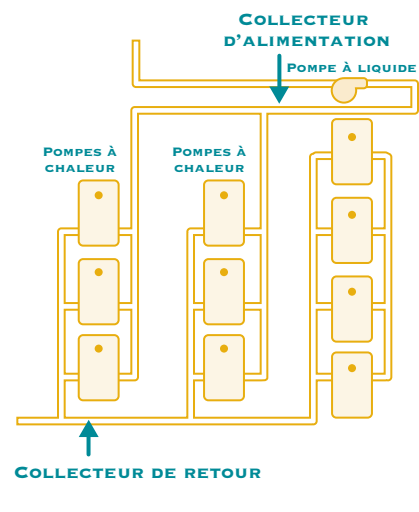
FIGURE 32. SYSTÈME À BOUCLE DE SOL
