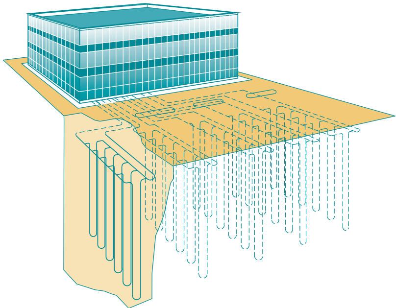
FIGURE 9. SYSTÈME À BOUCLE VERTICALE
