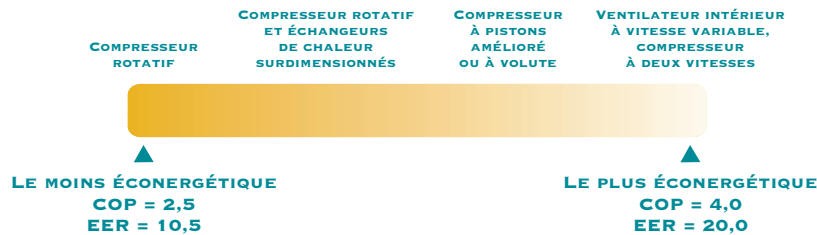
FIGURE 24. RENDEMENT DES SYSTÈMES À BOUCLE FERMÉE (À UNE TEMPÉRATURE D'EAU À L'ENTRÉE DE 10 °C)
