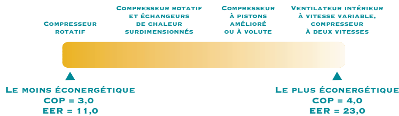
FIGURE 23. RENDEMENT DES SYSTÈMES À BOUCLE OUVERTE (À UNE TEMPÉRATURE D'EAU À L'ENTRÉE DE 10 °C)
