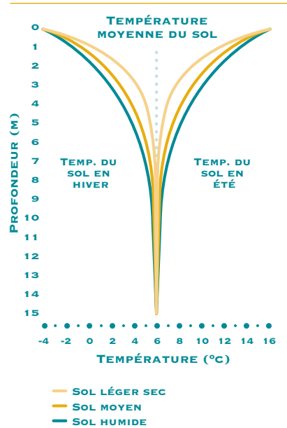
FIGURE 30. VARIATION DE LA TEMPÉRATURE DU SOL (°C)
