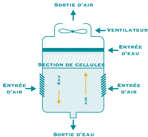
FIGURE 26. FONCTIONNEMENT DE LA TOUR DE REFROIDISSEMENT
