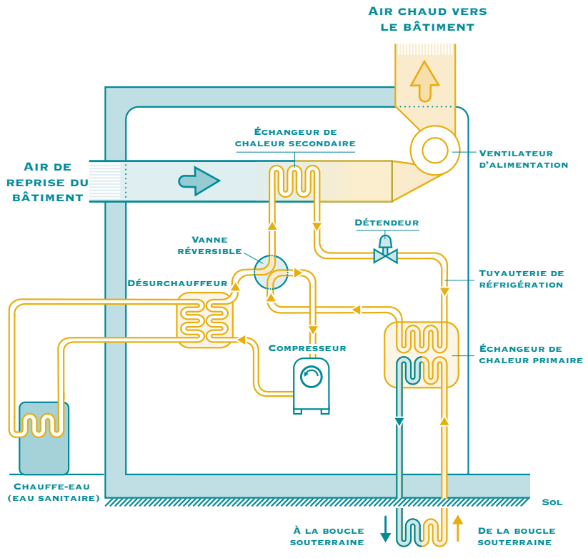
FIGURE 14. SCHÉMA SIMPLIFIÉ D'UNE POMPE À CHALEUR
