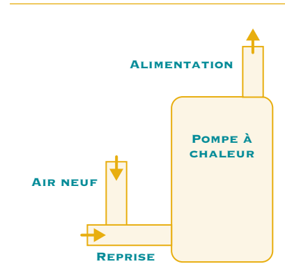
FIGURE 18. MÉLANGE D'AIR NEUF À LA POMPE À CHALEUR
