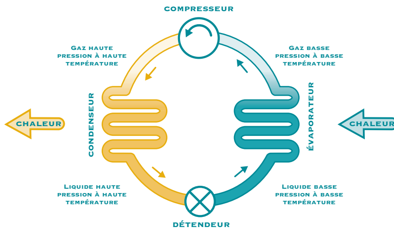
FIGURE 3. CYCLE DE RÉFRIGÉRATION (MODE CHAUFFAGE)
