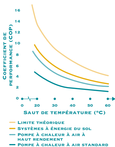
FIGURE 29. EFFET DU SAUT DE TEMPÉRATURE SUR LE RENDEMENT DES POMPES À CHALEUR
