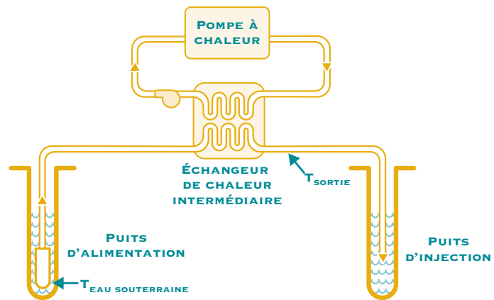
FIGURE 31. POMPE À CHALEUR À EAU SOUTERRAINE – SYSTÈME INDIRECT
